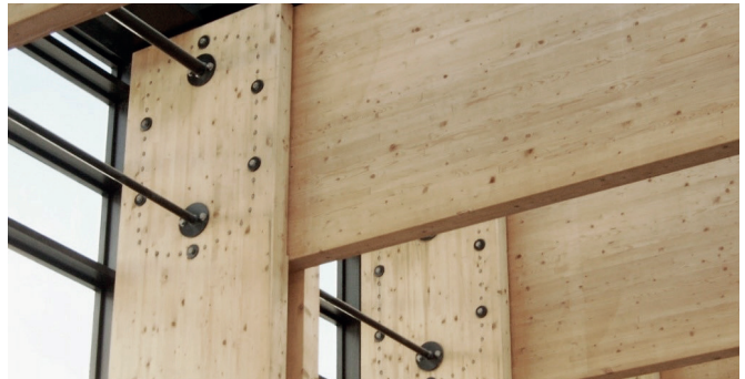
biegesteifes Rahmeneck mit rechteckigem Lichtraumprofil
