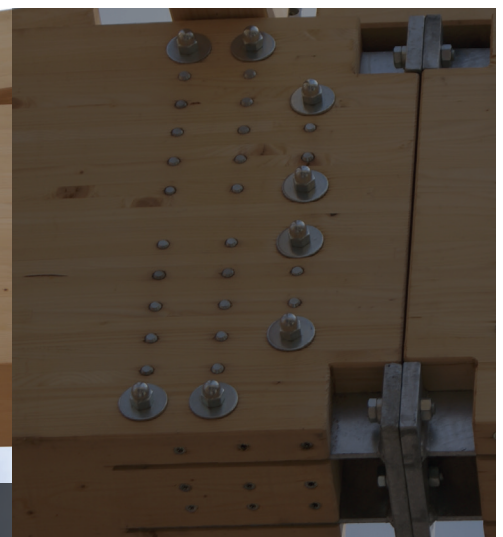
GVZ Ingolstadt Gleisüberdachung, unterspannte Bogenträger, komplette Vormontage im Werk
